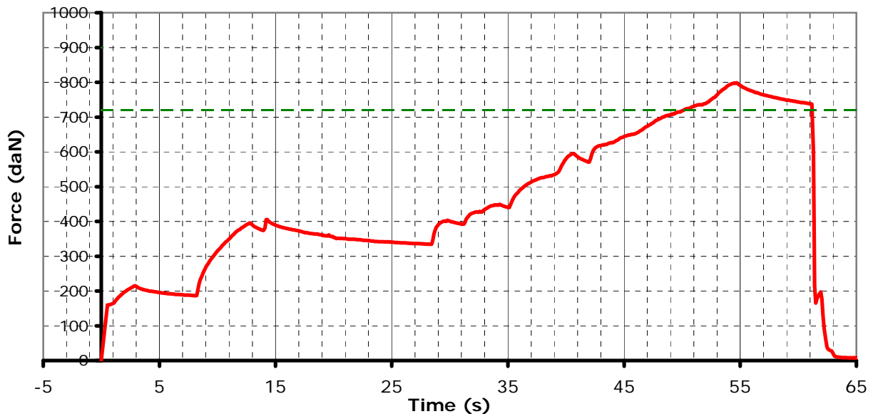
— TEST ID 1: EN 5.3.2.1 & LTF 4.2.1.a — — Norm 600 daN — — norm 900 daN
